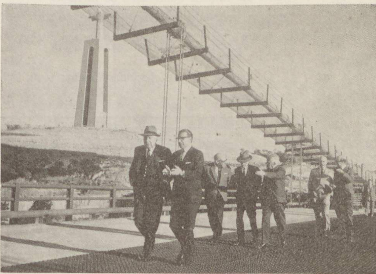
Durante a visita à Ponte — cuja construção, como se pode ajuizar por esta imagem, se encontra adiantadíssima — o sr. Prof. Mário de Figueiredo escuta atentamente as explicações do director do Gabinete da Ponte sobre o Tejo
