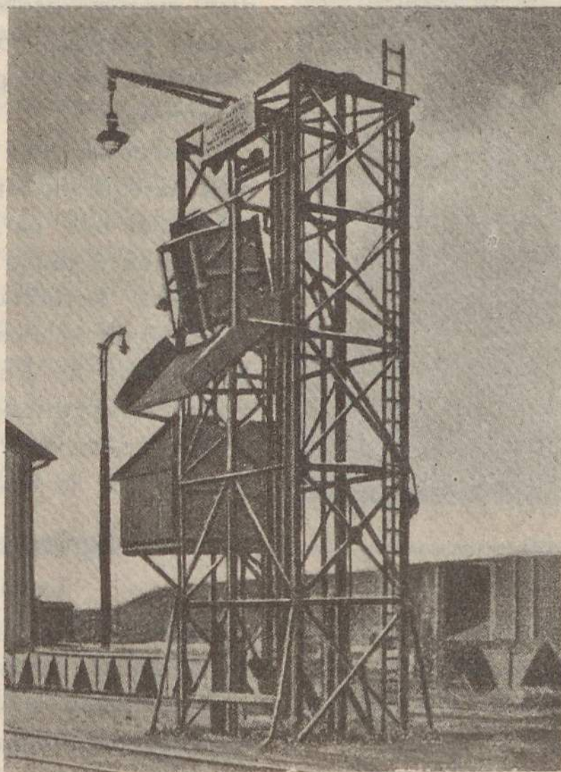
Fig. 1 — Aparelho elevador—descarregador
