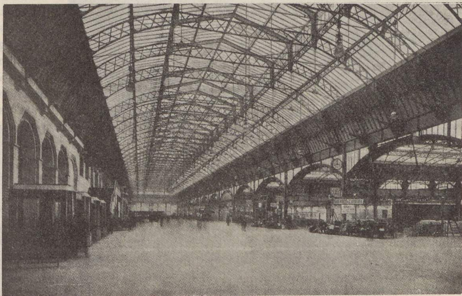
Fig. 3 — Cáis de tópo
