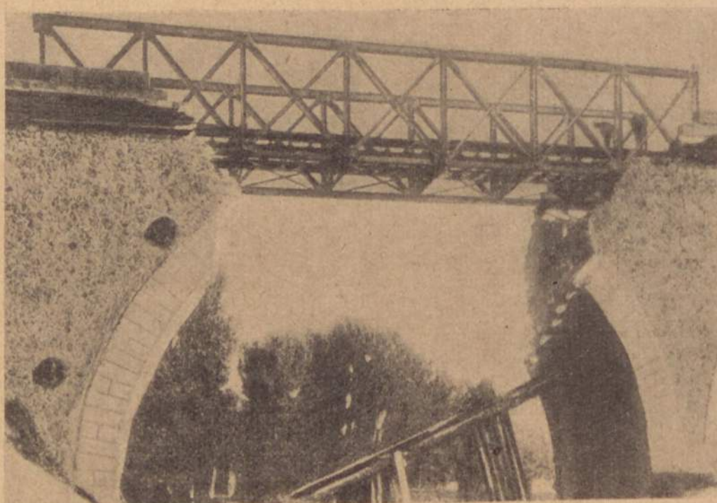
Os ingleses na Grande Guerra, durante a batalha do Marne, destruíram um dos arcos da ponte de Armentières, sobre o Marne, na linha férrea de Paris-Nancy, causando-lhe uma brecha de 17 m ,50 que teve de ser franqueada provisoriamente por uma ponte «Henry» de comprimento de 22 m ,80
