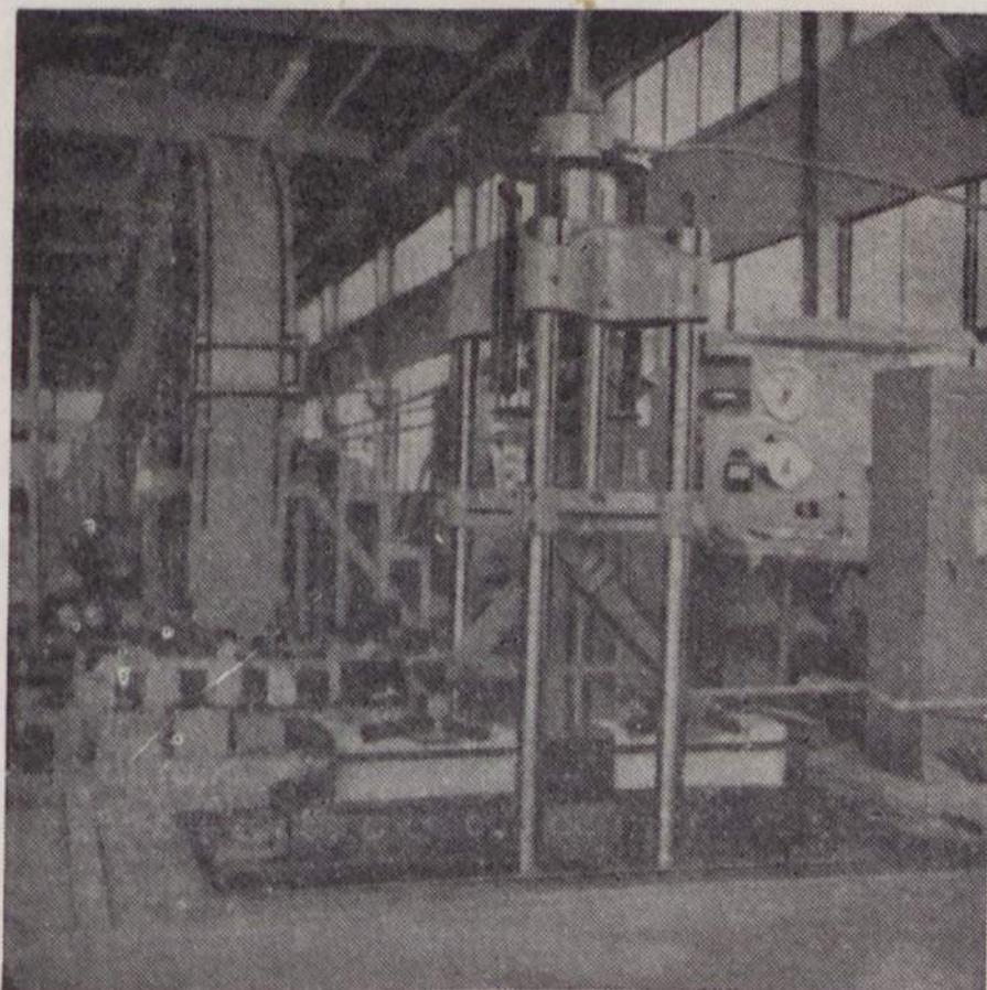
Máquina destinada a medir os esforços sofridos pelo carril
