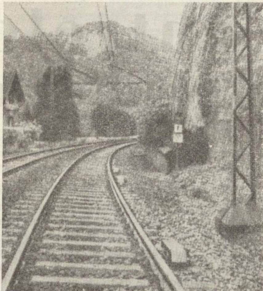
Instalação para o controlo de velocidade no troço perto de Geislingen. Por ordem, vê-se em primeiro plano o receptor de via, depois o íman de via, e logo o receptor de reposição. À direita a caixa de conexão.
