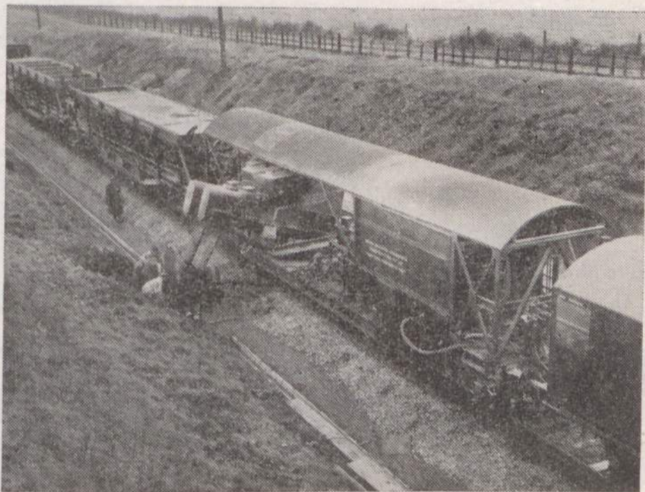
A electrificação de sistemas ferroviários requer uma perícia de elevadíssimo nível técnico e científico. Esta fotografia mostra um comboio utilizado na colocação do betão
