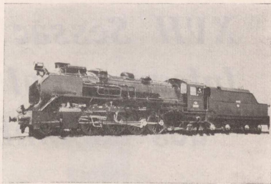
Locomotiva «Mikado» — Séries 141.2100. Anos 1.933/58, + 141.2200
