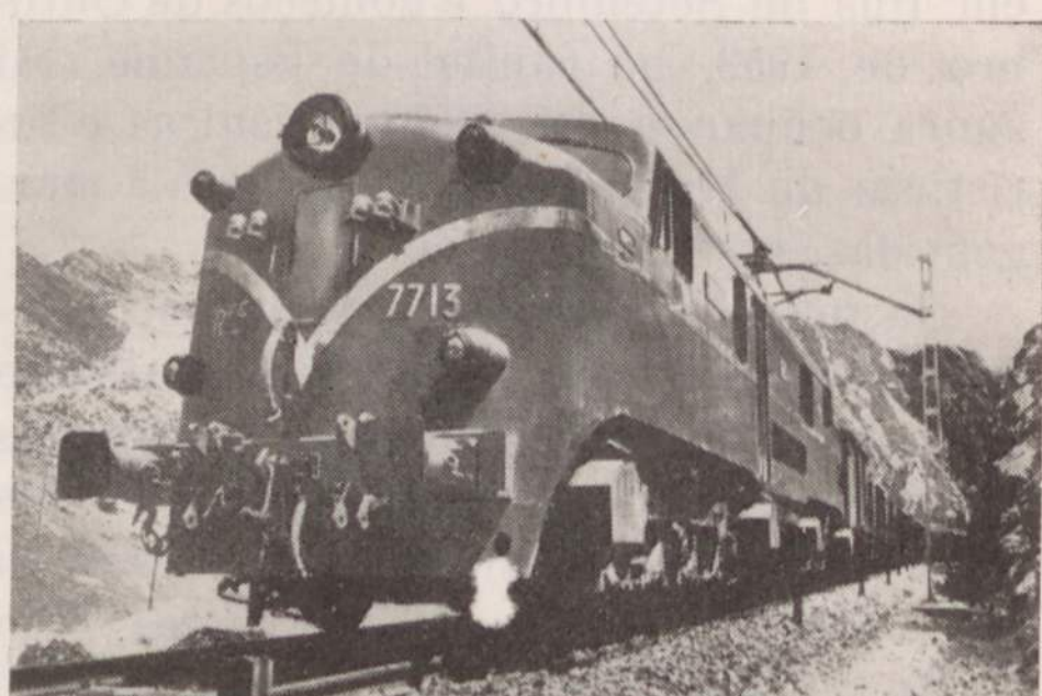
Locomotiva CoCo «English electric» — Série 7.700. Ano 1932.
