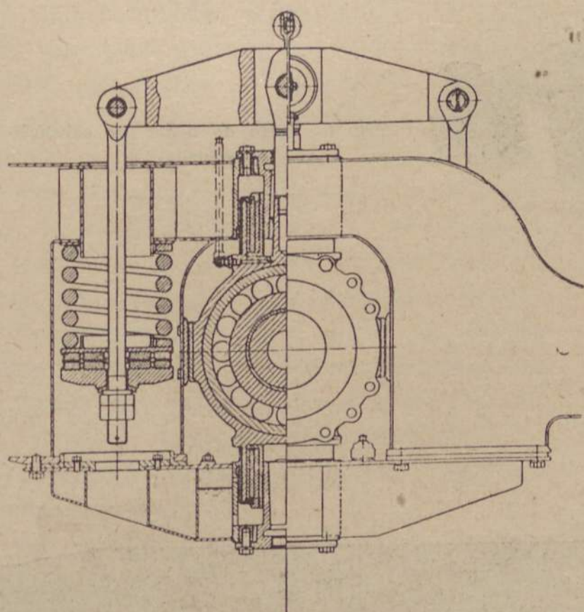
Fig. 2 - Caixas de lubrificação com munhões de guia cilíndricos
