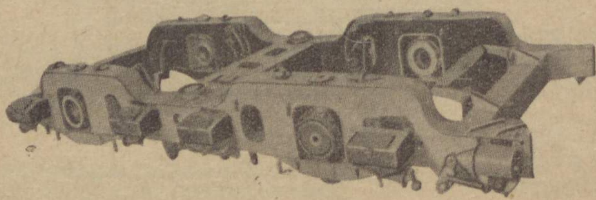
Fig. 4 — leito do bogie com as caixas de lubrificação incorporadas
