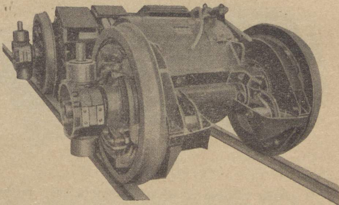
Fig. 3 - Caixa de lubrificação
