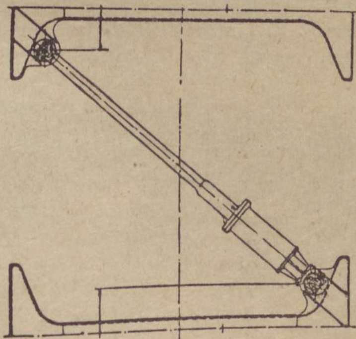
Fig. 7 - Disposição do acoplamento diagonal
