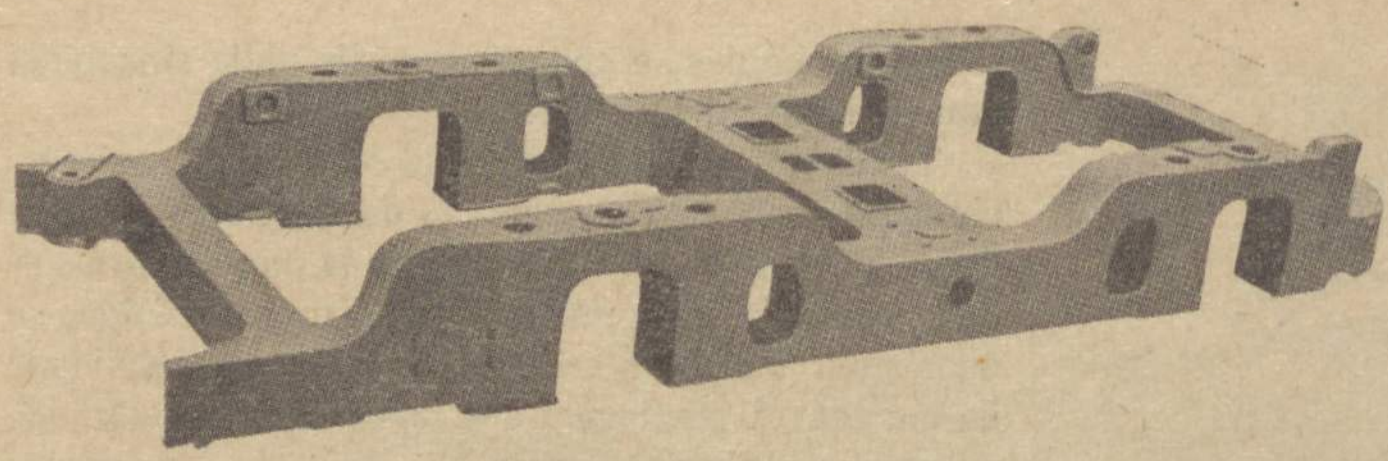
Fig. 1 — Leito do bogie (de execução soldada)
