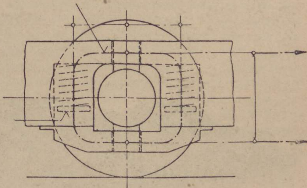
Fig. 5 - Guia de caixa de lubrificação com munhões dispostos um por cima do outro
