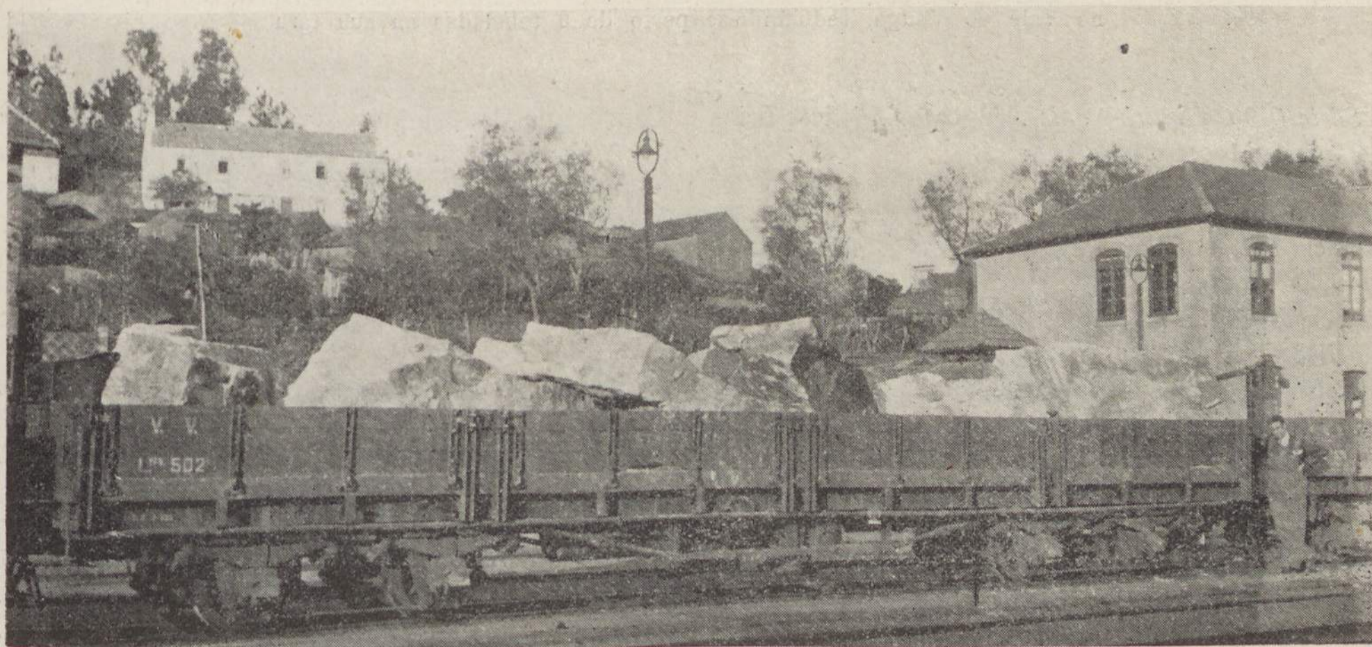
Vagão de 30 toneladas, antigo auto-descarregador do Lena, reconstruído e transformado nas oficinas do Vale do Vouga, na Sernada
