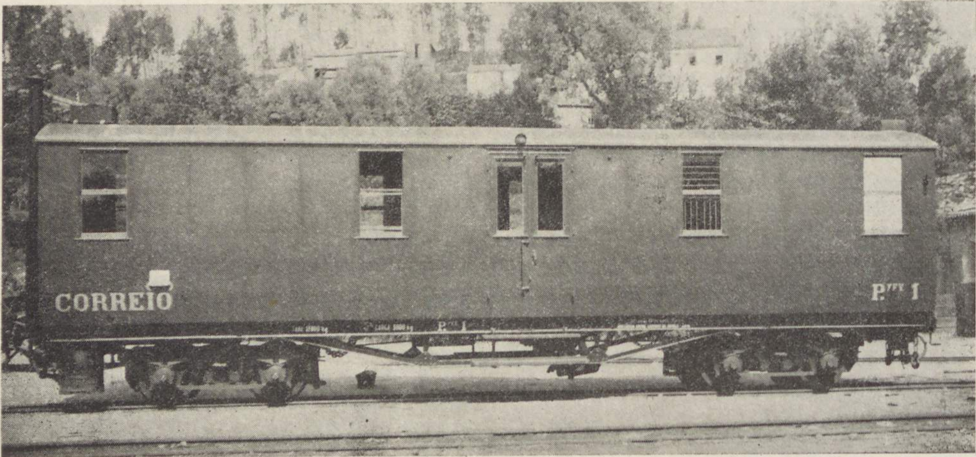
Ambulância postal adquirida pelas «Reparações Alemãs» e reconstruída no Vale do Vouga, reduzindo-se perto de 3 toneladas na sua tara
